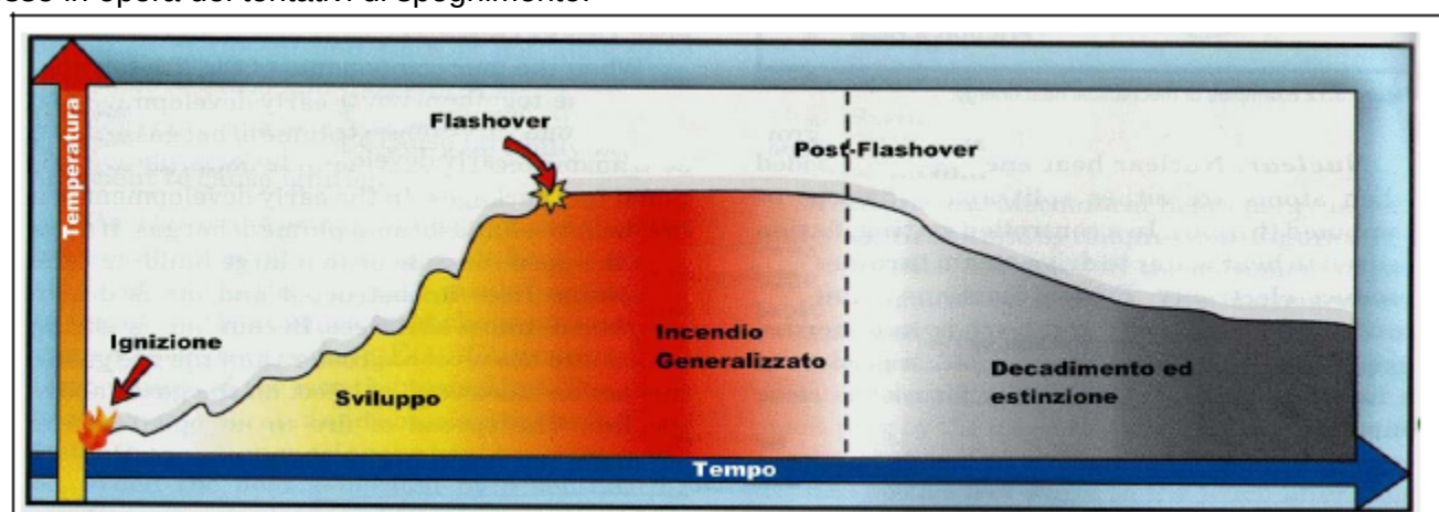
Fig. 7 – Grafico incendio in funzione temperatura/tempo
